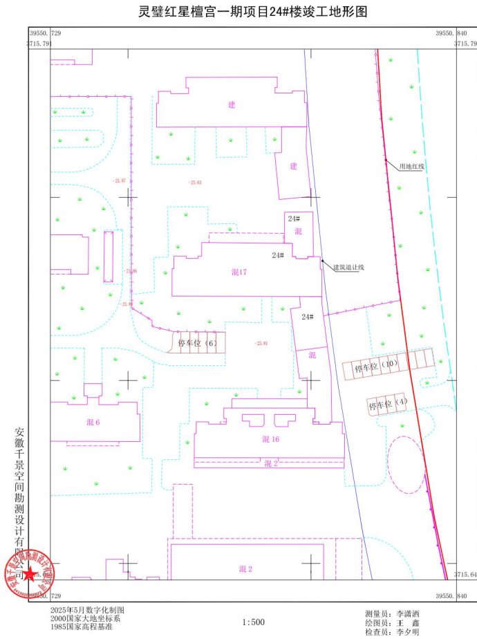
现竣工验收图
