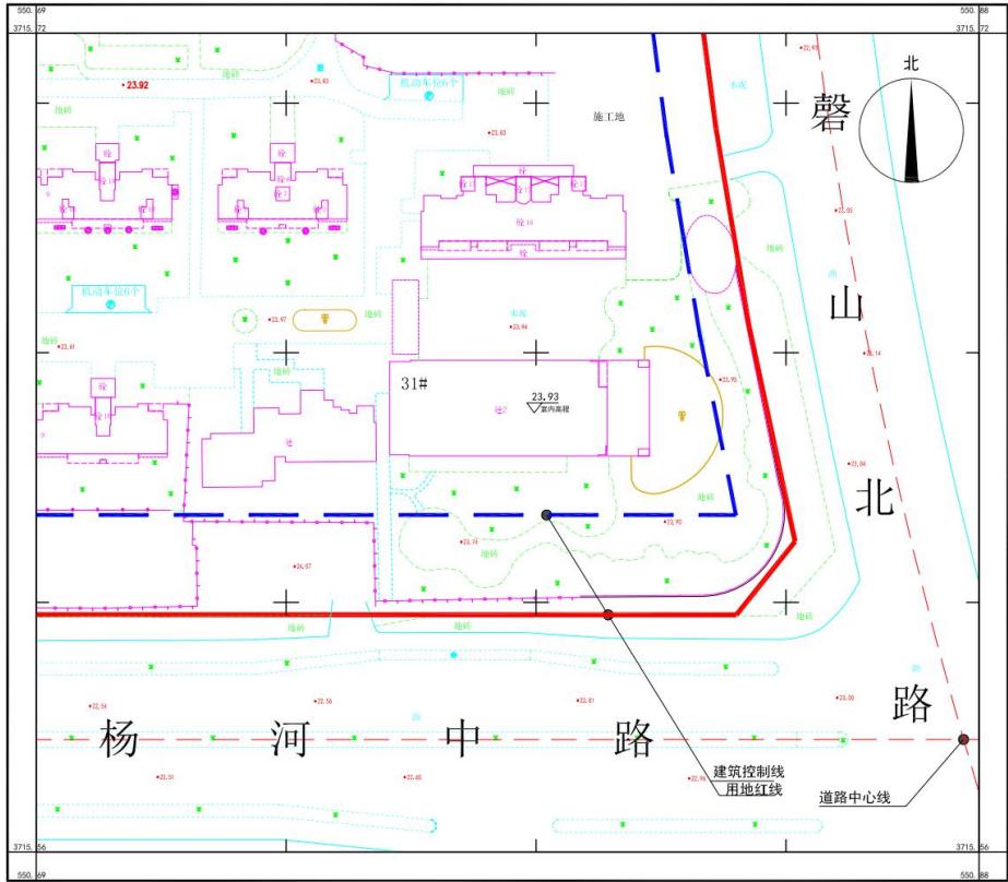
灵璧红星檀宫一期项目(31#)竣工总平图 3715.557-550.691
