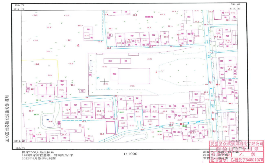
竣工总平面图
