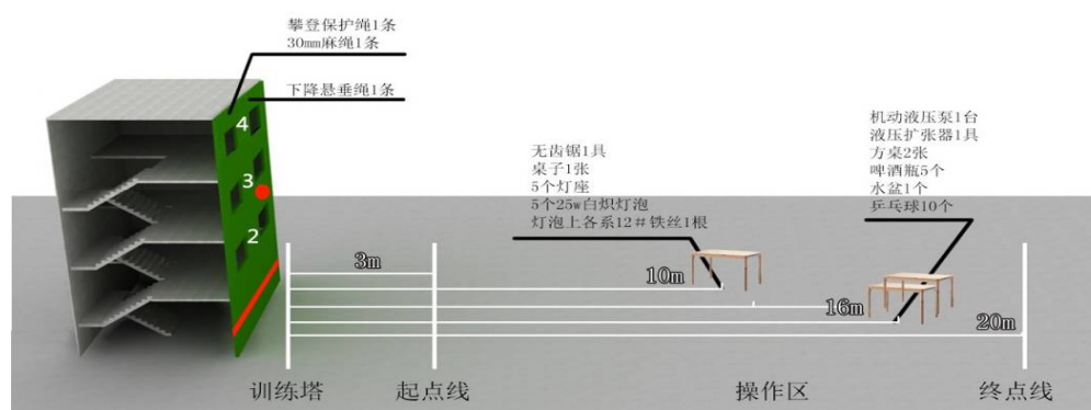
图 3 攻坚技巧场地器材设置示意图
