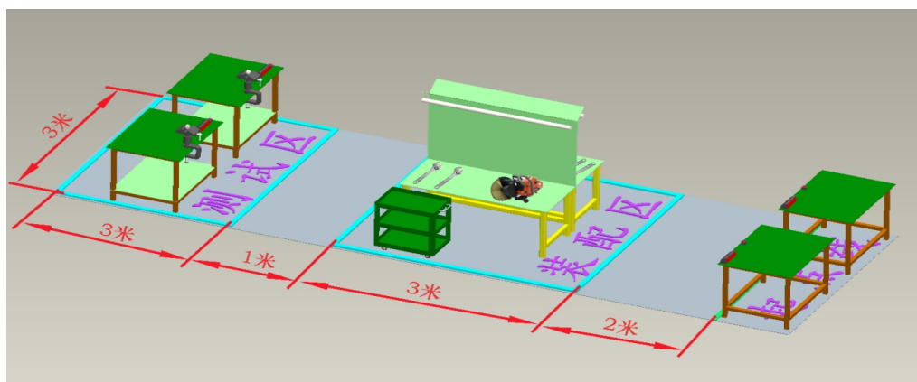
图 2 双轮异向切割锯（机动）组装及应用场地示意图
