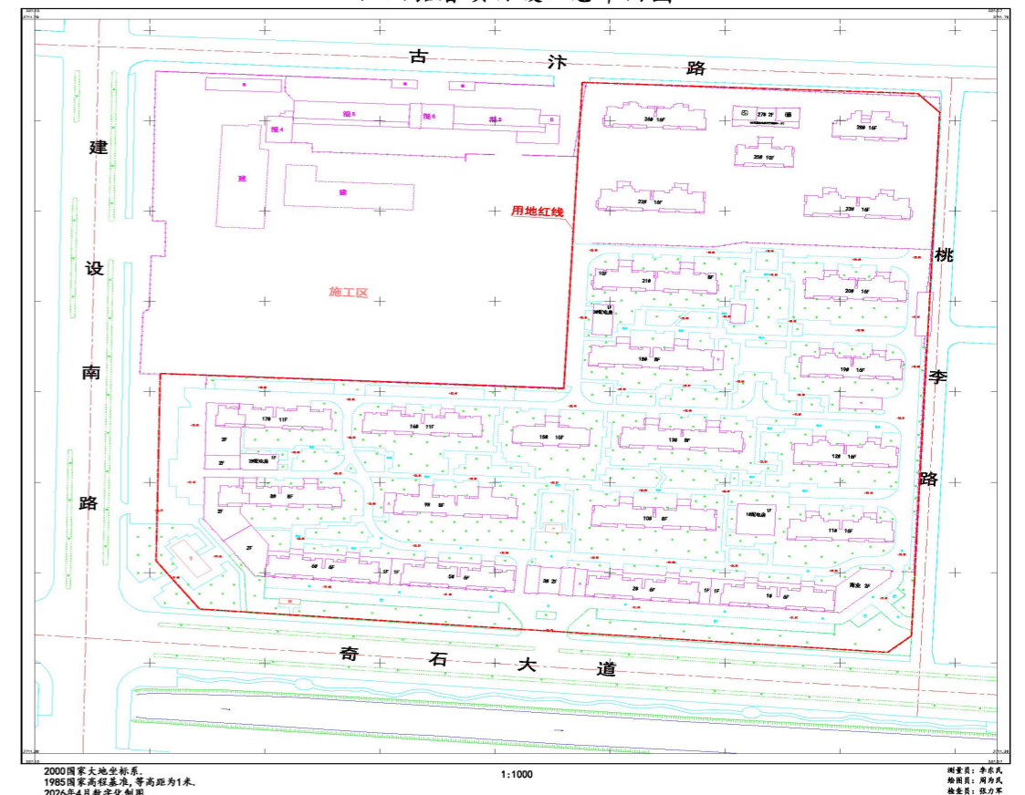
江山铭著项目竣工总平面图
